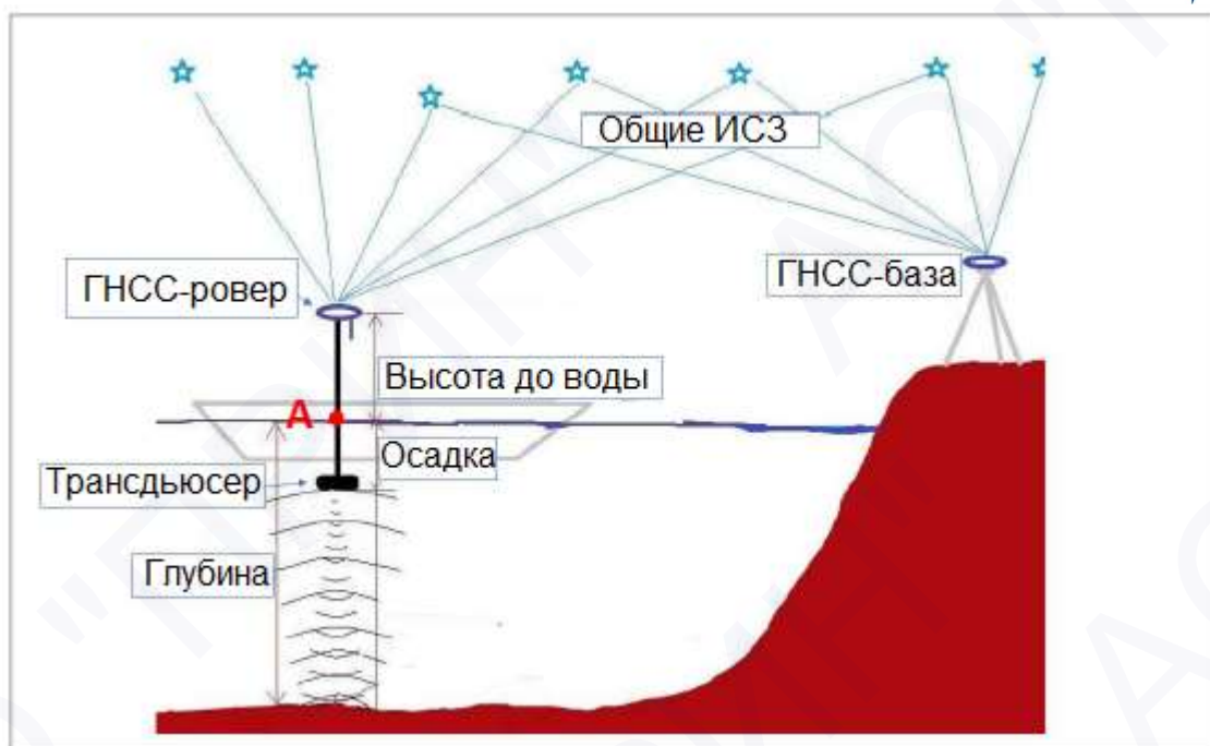
Рис. 2.1 Принцип съёмки глубин с использованием эхолота и RTK приёмника
