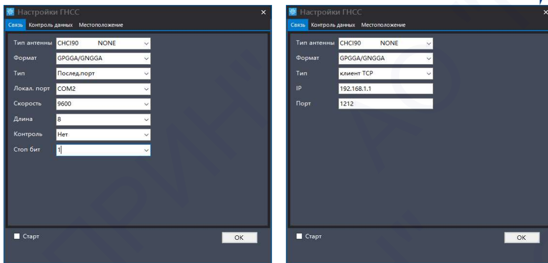
Рис. 4.6 Настройка связи с ГНСС-приёмником
