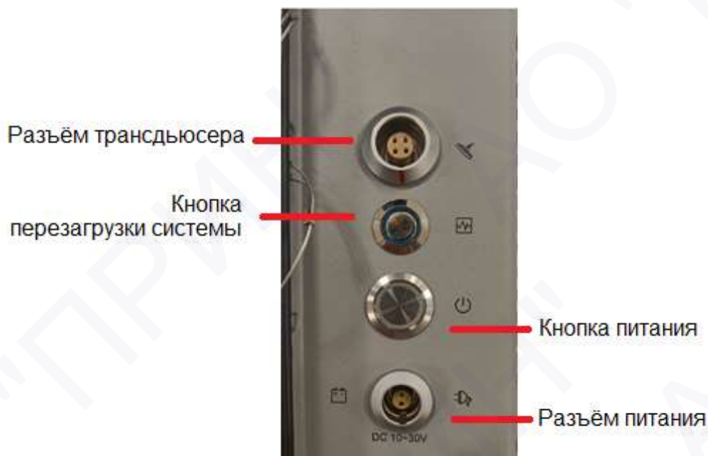
Рис. 2.3 Разъёмы на правой стороне
