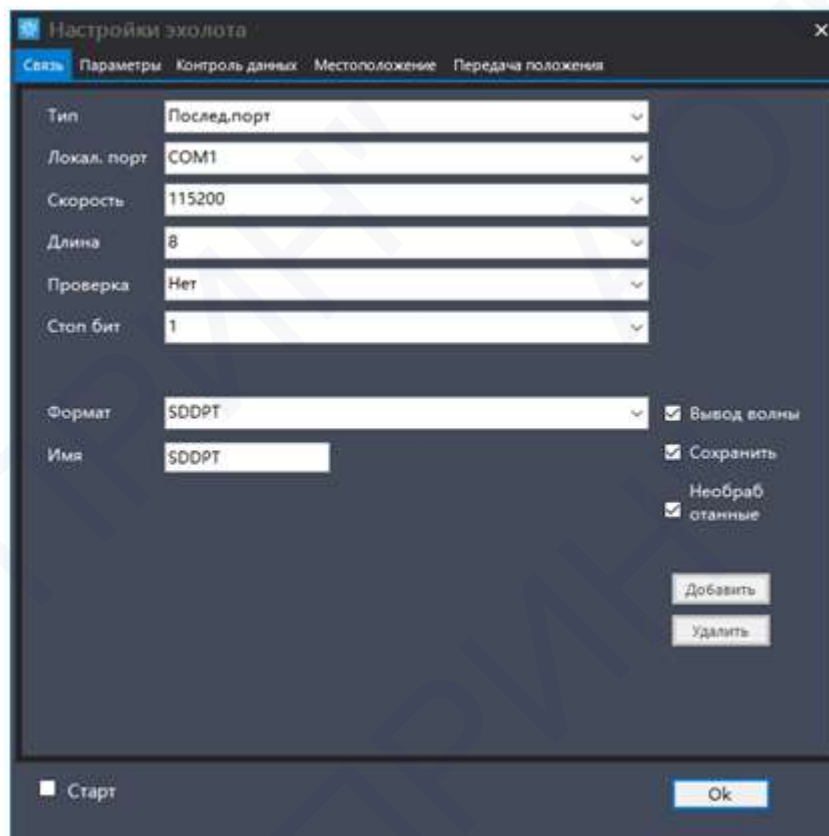
Рис. 4.3. Настройка связи с эхолотом
