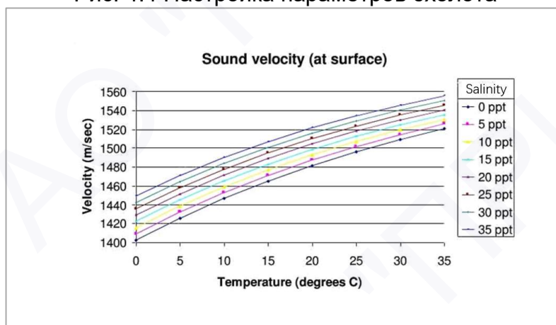
Рис. 4.5 Зависимость скорости звука в воде от температуры и солёности
