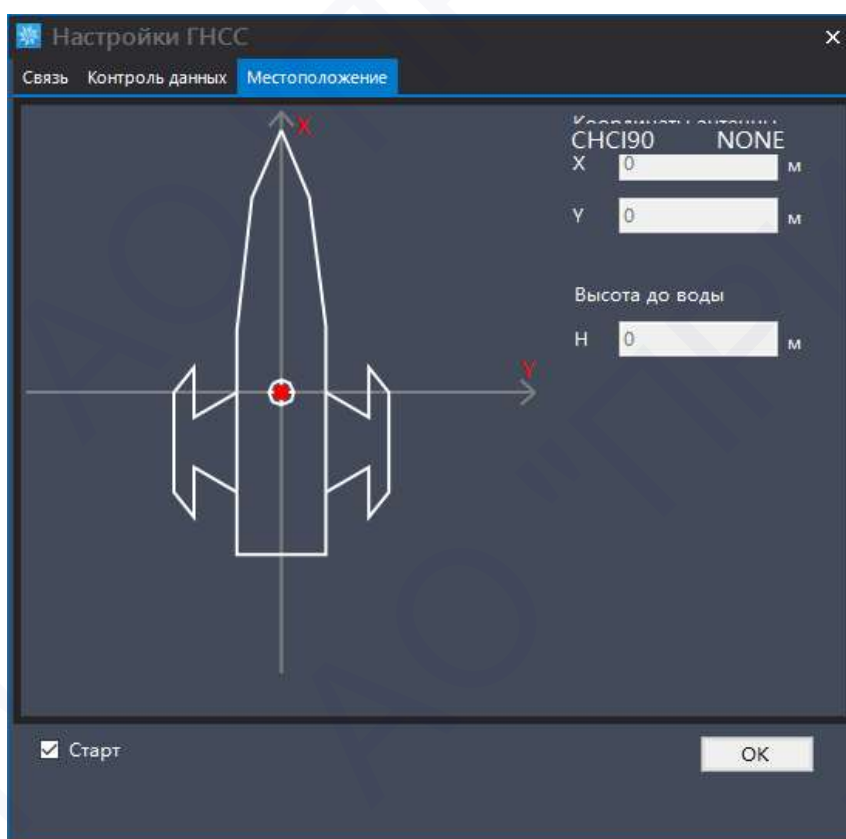
Рис. 4.7 Настройка параметров местоположения ГНСС-приёмника
