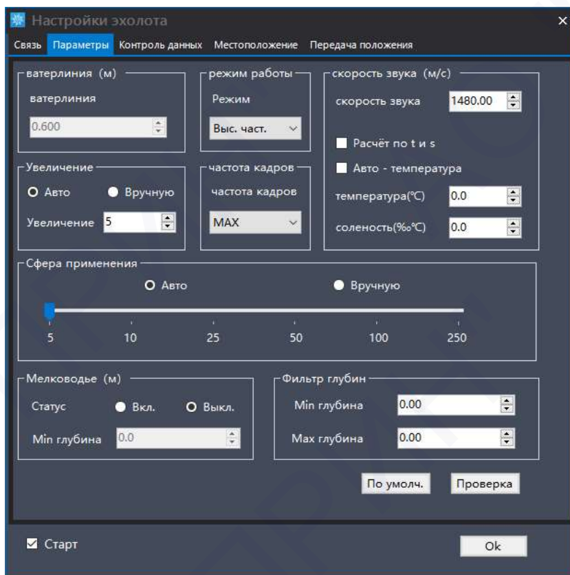
Рис. 4.4 Настройка параметров эхолота
